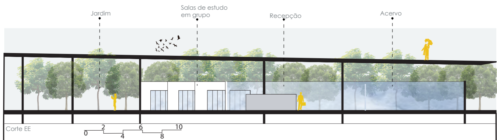
Corte EE
