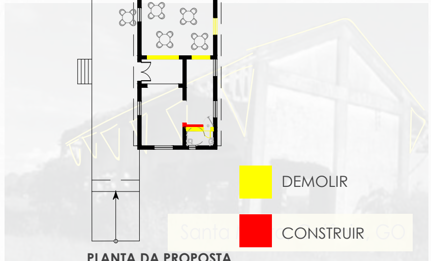
PLANTA DA PROPOSTA (CAFETERIA E MUSEU FOTOGRÁFICO)
